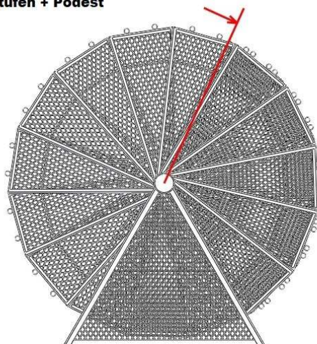
20 Stufen + Podest
