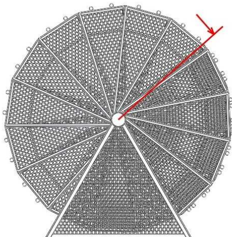
19 Stufen + Podest
