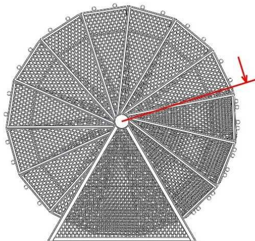
18 Stufen + Podest
