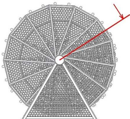
17 Stufen + Podest
