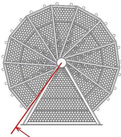
13 Stufen + Podest
