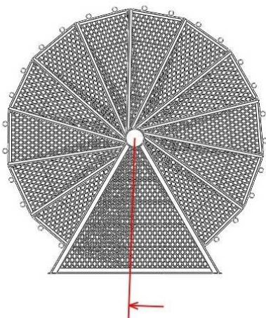
15 Stufen + Podest
